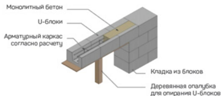
Схема изготовления перемычки из U-блоков «ЭКО»
