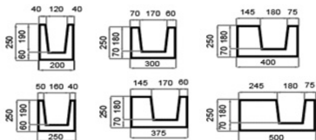
Схема изготовления U-блоков «ЭКО»
