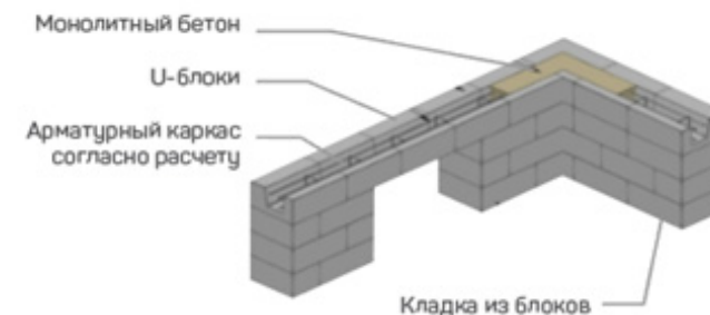
Схема изготовления армопояса из U-блоков «ЭКО»
